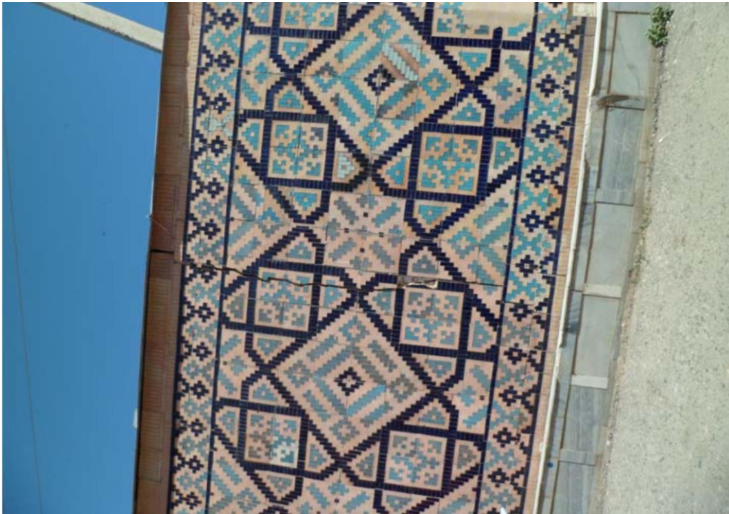
Фото 7 б. Поперечные трещины на изразцах портала мавзолея Гур-Эмир, г. Самарканд, 2013 г. (фото Усмановой М.Т.)
