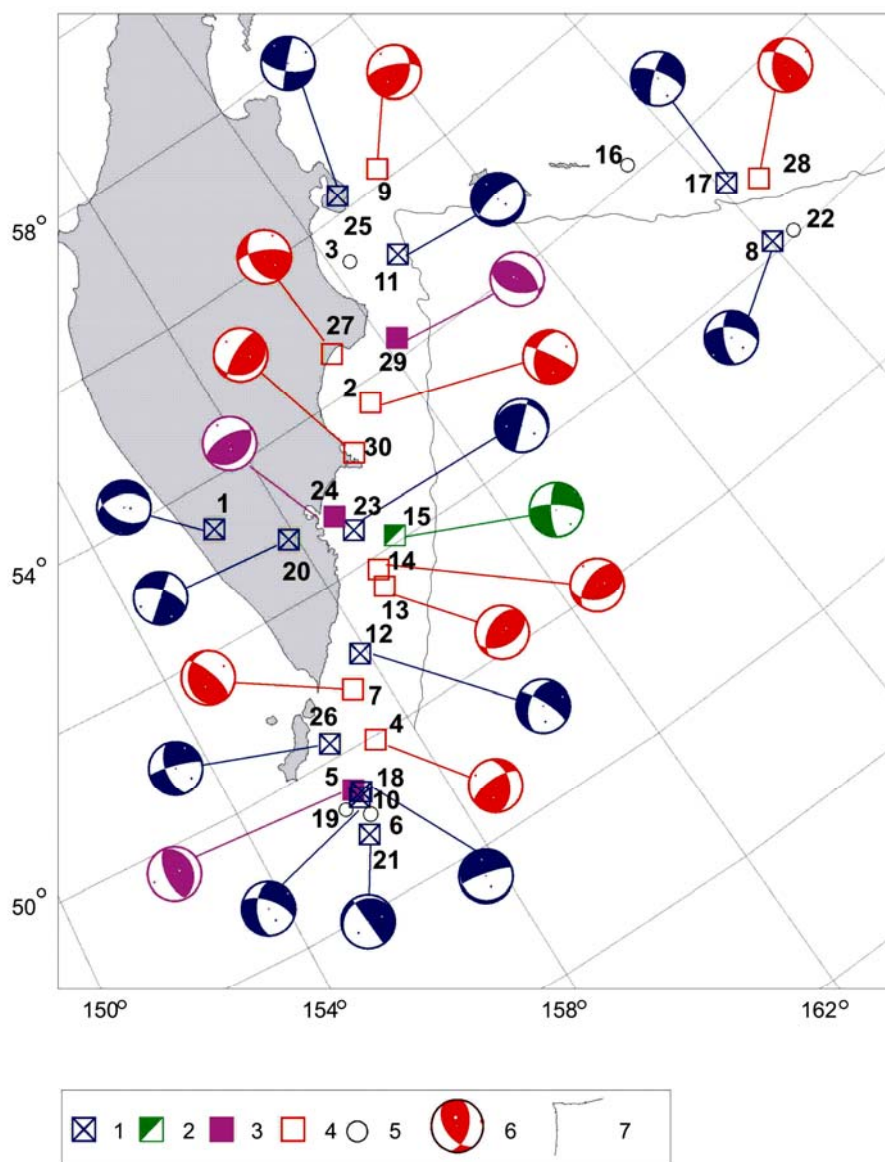
Рис. 4. Карта эпицентров сильных K_S \geq 11.6 землетрясений Камчатки и Командорских островов за 2000 г. 1–5 – эпицентры землетрясений и тип подвижки (1 – сбросо-сдвиг; 2 – сдвиг; 3 – взброс; 4 – взбросо-сдвиг; 5 – механизм не определен); 6 – диаграмма механизма очага; 7 – изобата морских глубин, 5000 м. Числа возле эпицентров соответствуют номерам землетрясений первой графы каталога [5].
