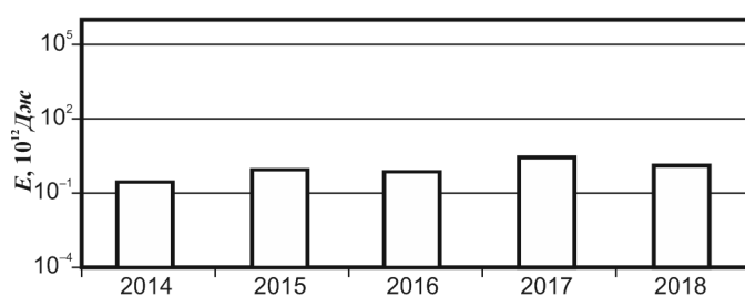
Рис. 1.12. Распределение сейсмической энергии, выделившейся в районе Арктики в 2014–2018 гг.
