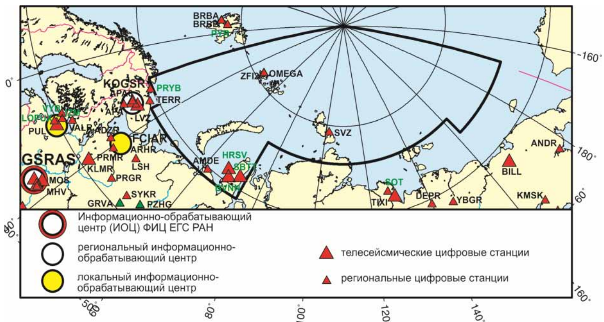
Рис. I.10. Сейсмические станции Арктического региона и севера РФ в 2018 г.
