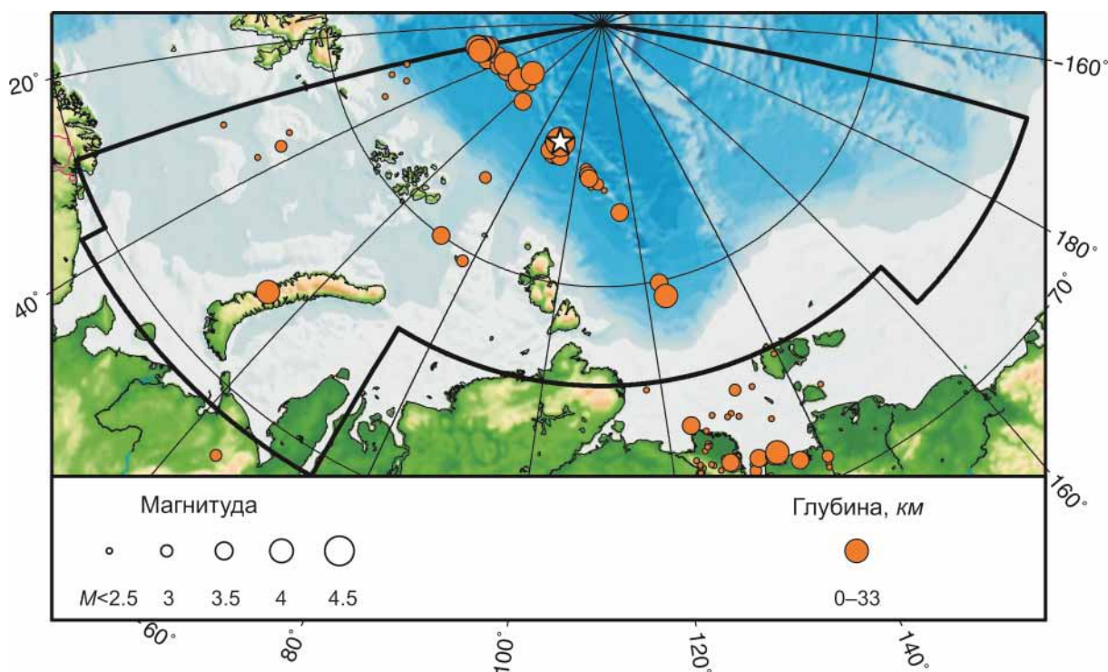
Рис. I.11. Карта эпицентров землетрясений в районе Арктики в 2018 г.
