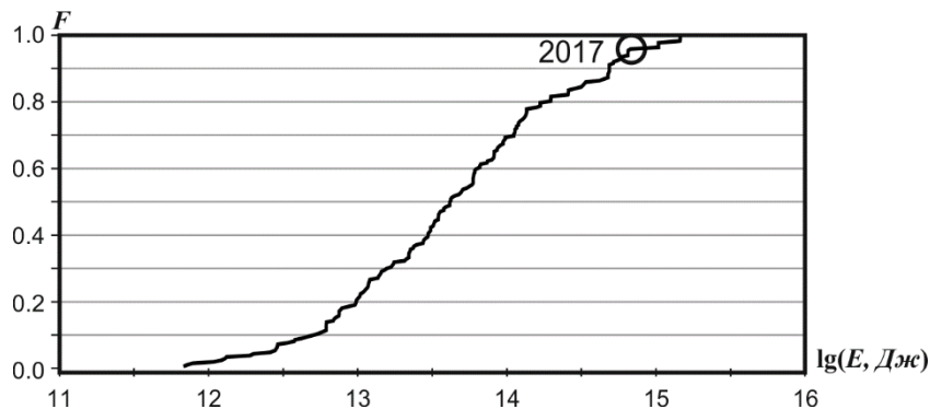
Рис. II.3. Функция распределения сейсмической энергии для региона Арктика
