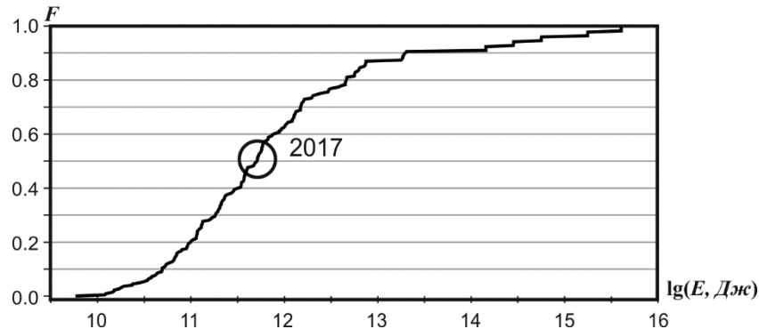
Рис. II.7. Функция распределения сейсмической энергии для региона Сахалин
