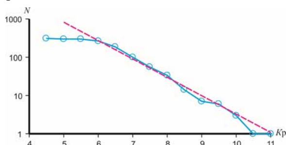
Рис. III.10. Кумулятивный график повторяемости землетрясений: \gamma=0.48 , K_{pmin}=6.5
