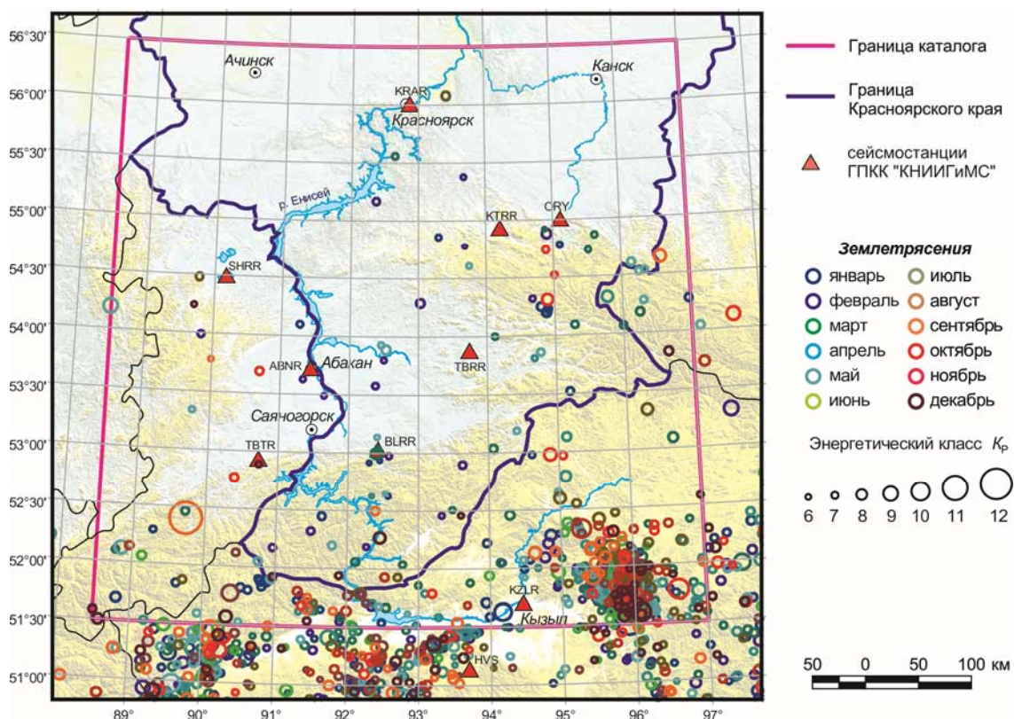
Рис. III.9. Сейсмические станции ГПКК «КНИИГиМС» и эпицентры землетрясений центральных и южных районов Красноярского края в 2015 г.
