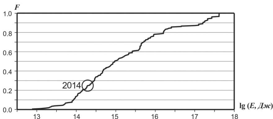
Рис. П.8. Функция распределения сейсмической энергии для Курило-Охотского региона
