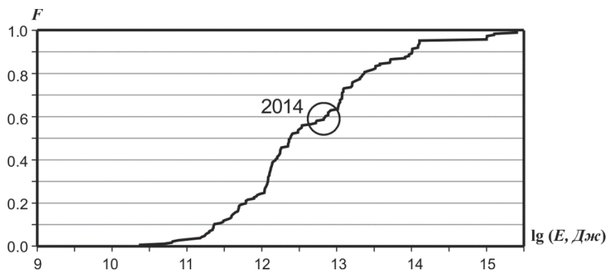
Рис. II.10. Функция распределения сейсмической энергии для региона Северо-Востока России и Чукотки
