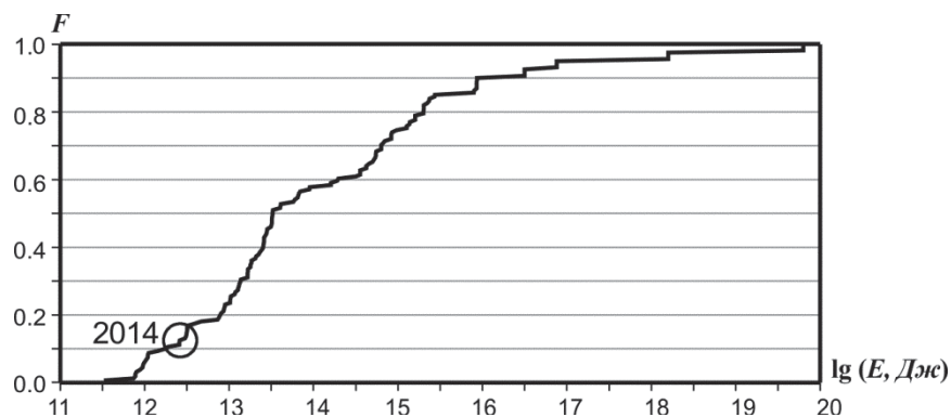
Рис. II.6. Функция распределения сейсмической энергии для региона Приамурья и Приморья
