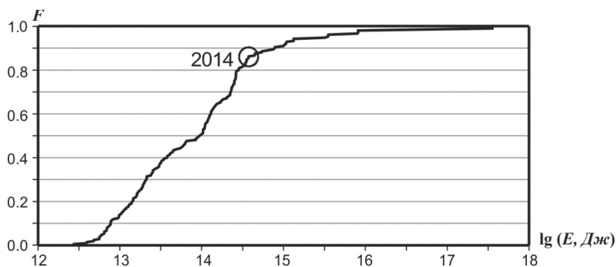
Рис. II.5. Функция распределения сейсмической энергии для региона Прибайкалья и Забайкалья
