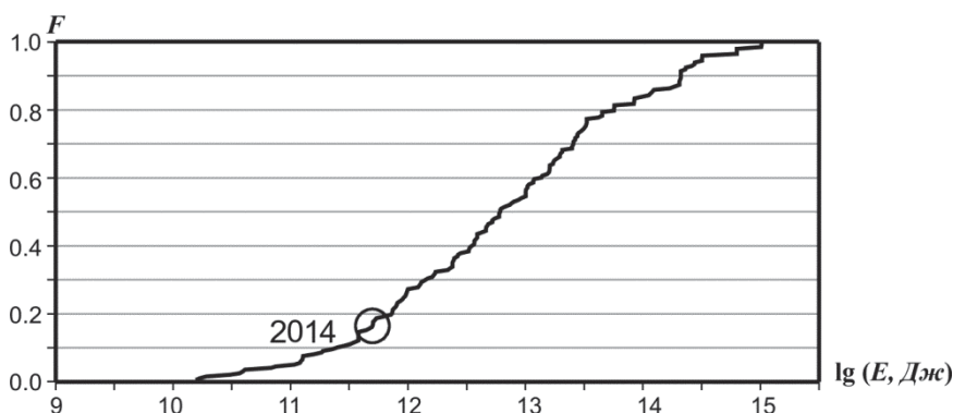
Рис. II.3. Функция распределения сейсмической энергии для региона Арктики
