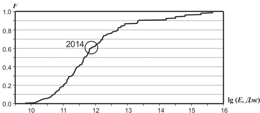
Рис. П.7. Функция распределения сейсмической энергии для региона Сахалина
