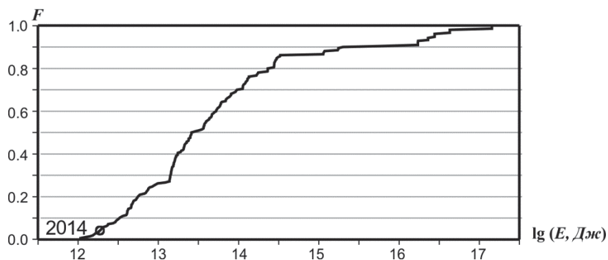
Рис. II.4. Функция распределения сейсмической энергии для региона Алтая и Саян
