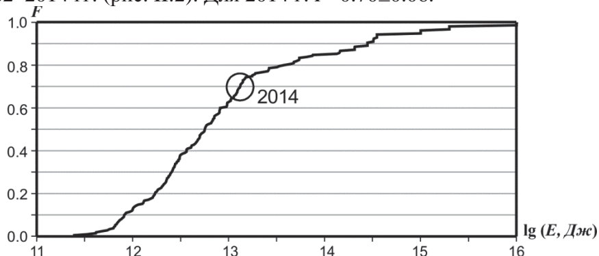
Рис. II.2. Функция распределения сейсмической энергии для региона Северного Кавказа
