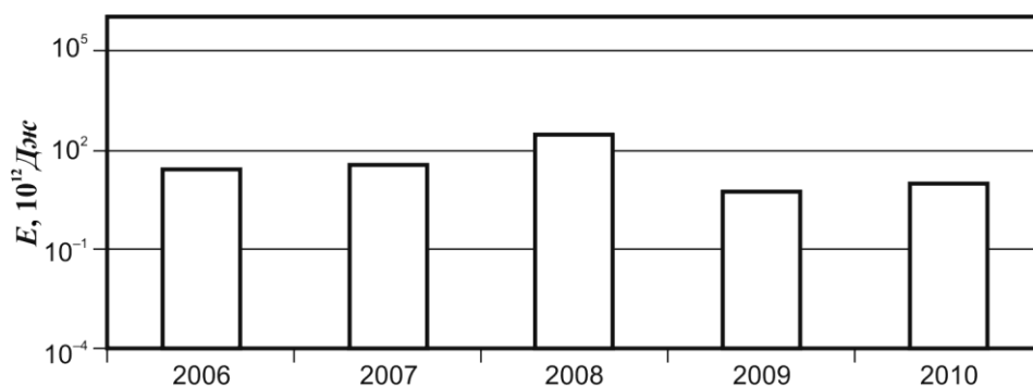
Рис. I.17. Гистограмма распределения сейсмической энергии, выделившейся в регионе Прибайкалья и Забайкалья в 2006–2010 гг.
