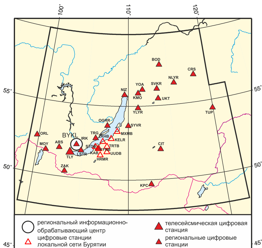
Рис. 1.15. Сейсмические станции в Прибайкалье и Забайкалье в 2010 г.: Черный шрифт – международные коды сети (центра) и станций
