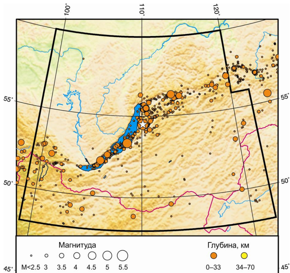
Рис. 1.16. Карта эпицентров землетрясений Прибайкалья и Забайкалья в 2010 г. Звездочкой показано самое сильное землетрясение в регионе
