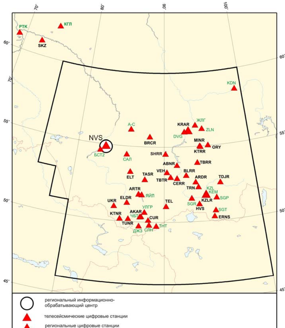
Рис. 1.12. Стационарные сейсмические станции в Алтае-Саянском регионе в 2007 г.
