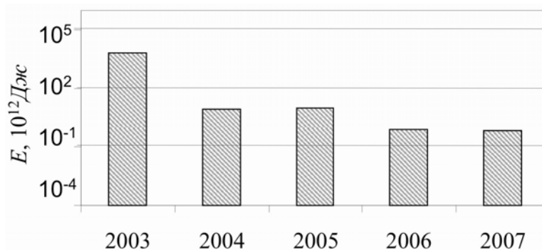
Рис. 1.14. Гистограмма распределения сейсмической энергии, выделившейся в Алтае-Саянском регионе в 2003–2007 гг.
