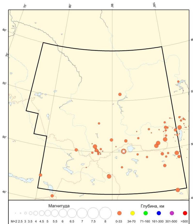
Рис. 1.13. Карта эпицентров землетрясений в Алтае-Саянском регионе в 2007 г.
